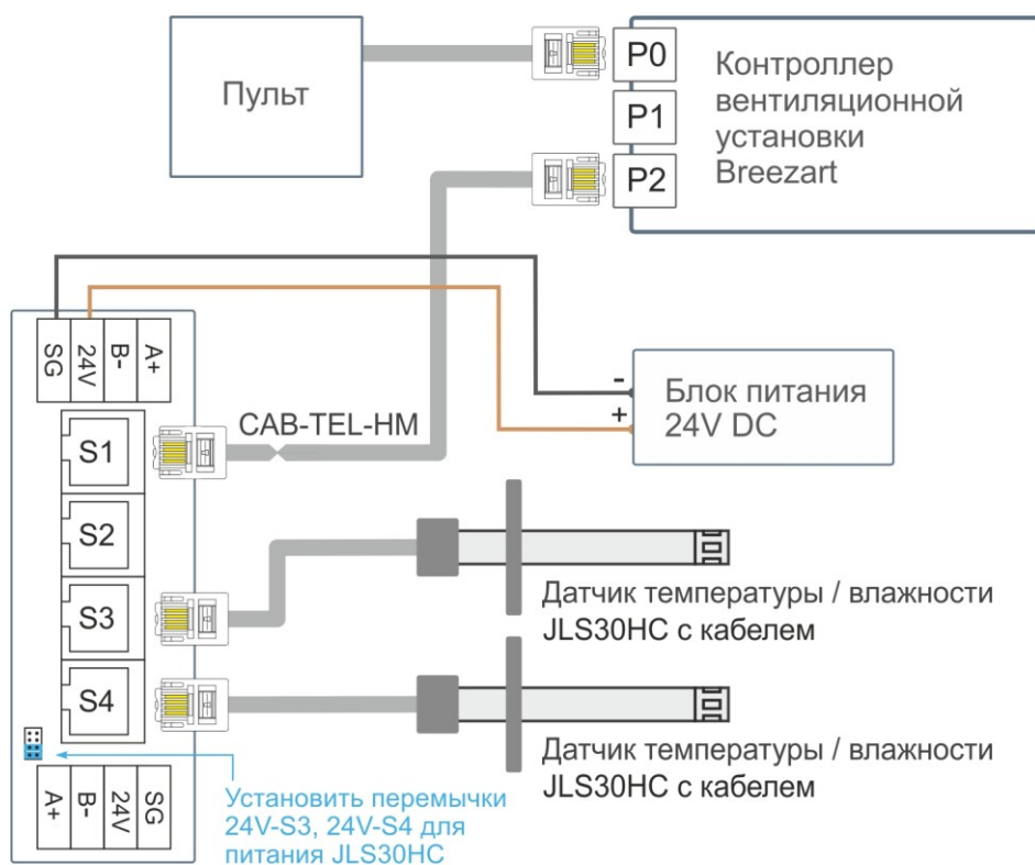
Кроссовый модуль RSCON-03
